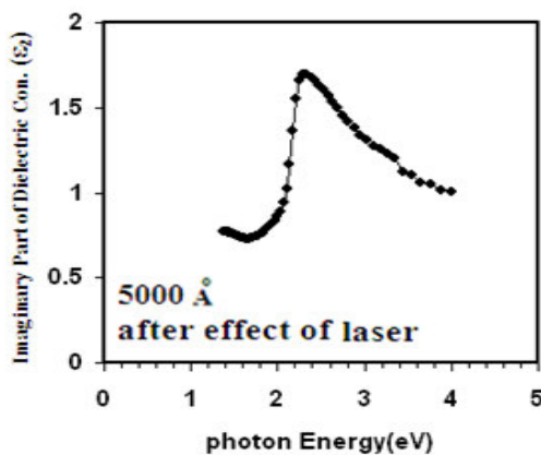
الشكل (8) الجزء الخيالي لثابت العزل الكهربائي كدالة لطاقة الفوتون للأغشية المحضرة بأسماك مختلفة قبل وبعد المعاملة الليزر
