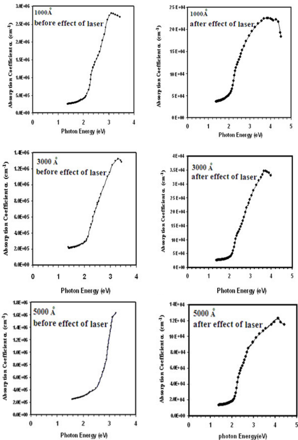
الشكل (3) يبين معامل الامتصاص كدالة لطاقة الفوتون للأغشية المحضرة بأسماك مختلفة قبل وبعد المعاملة الليزرية
