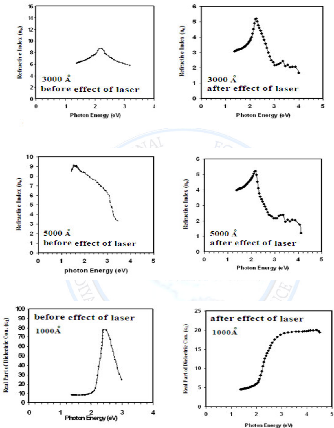
الشكل (6) يبين معامل الانكسار كدالة لطاقة الفوتون للأغشية المحضرة بأسماك مختلفة قبل وبعد المعاملة الليزر
