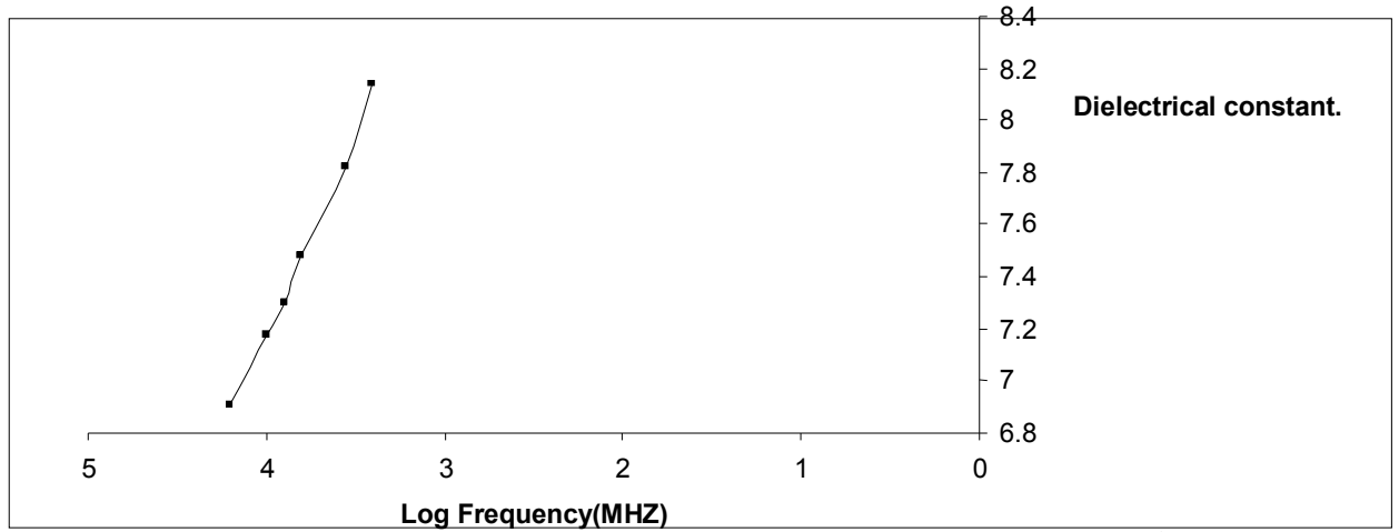
شكل (٤) : يوضح تأثير اشعة ليزر النيديميوم زجاج على مقدار التغير الحاصل في مقدار قيمة ثابت العزل الكهربائي للنموذج C بطاقة
