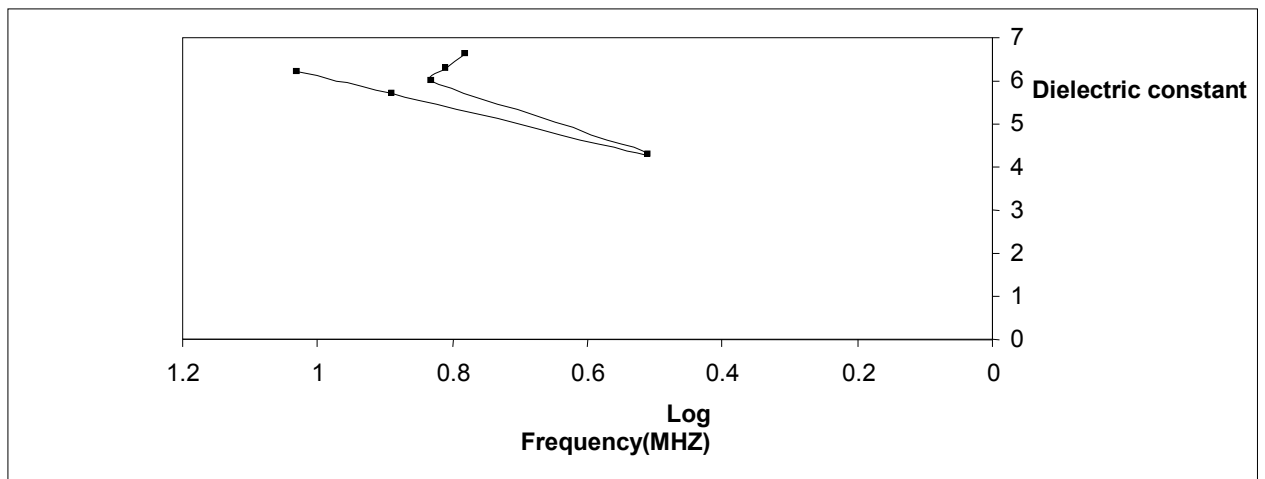
شكل (٥) : يوضح تأثير اشعة ليزر النيديميوم زجاج على مقدار التغير الحاصل في مقدار قيمة ثابت العزل الكهربائي
