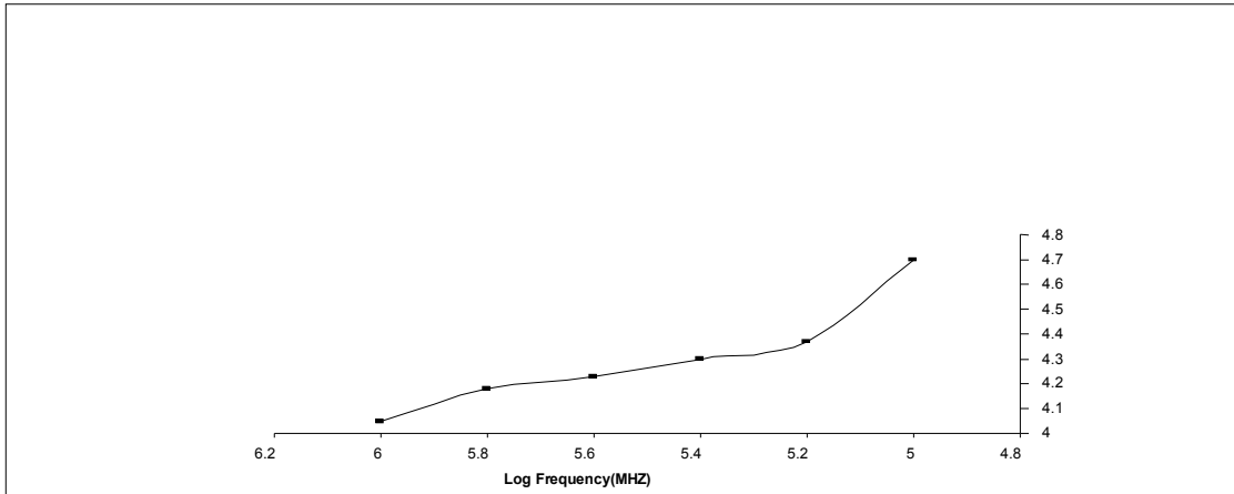
شكل (١): يوضح مقدار التغير الحاصل في مقدار قيمة ثابت العزل الكهربائي للنموذج السيراميكي A
