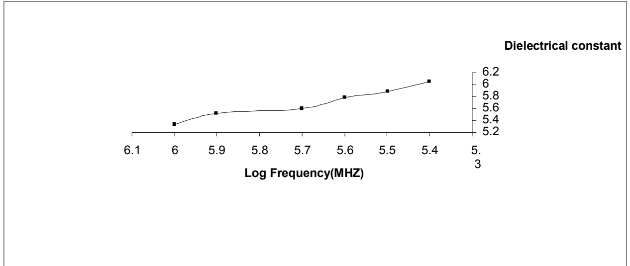
شكل (٣) : يوضح مقدار التغير الحاصل في مقدار قيمة ثابت العزل الكهربائي للنموذج C
