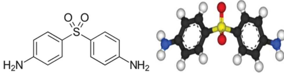
شكل (٣-١) تركيب الدابسون
