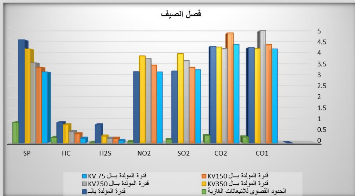
الشكل (٢) معدل تحليل الانبعاثات الغازية عن المولدات الاهلية
